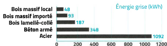
ÉNERGIE NÉCESSAIRE POUR LA FABRICATION DE DIFFÉRENTS MATÉRIAUX (pour une poutre de 3 mètres supportant 3 tonnes)
